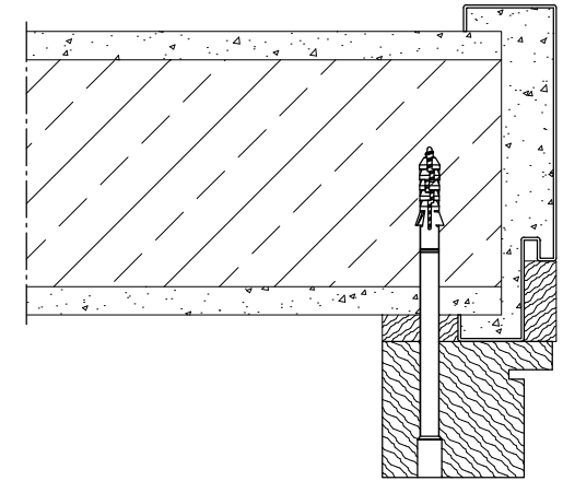
Sanierungsmöglichkeit 1: Holzblendrahmenelement über bestehende Stahlzarge montiert
